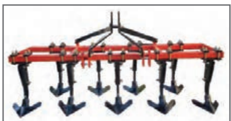
شکل ۲۰- گاو آهن پنجه‌غازی
