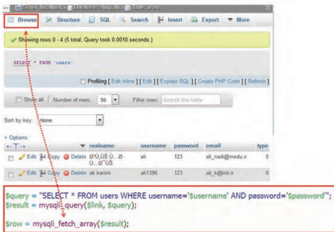
شکل ۴۸- عملیات معادل تابع mysqli_fetch_array در phpMyAdmin
