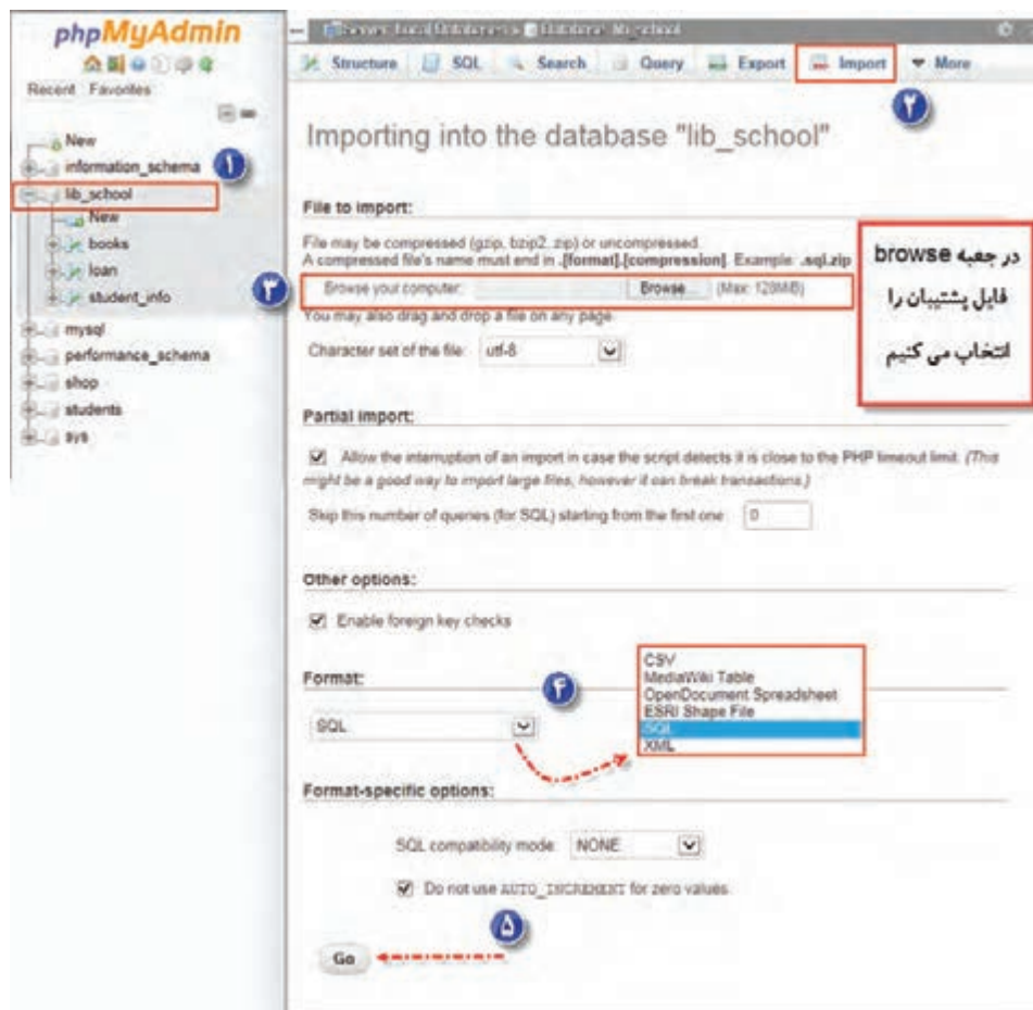
شکل ۵۴- انتخاب پرونده پشتیبان
