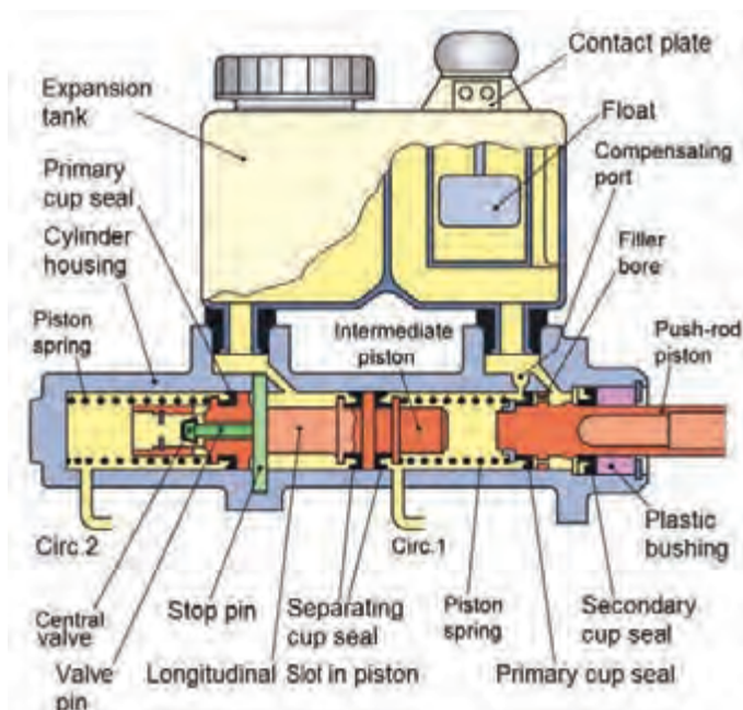
ترمز سیلندر اصلی
