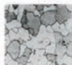
0.1 % C فرویت
