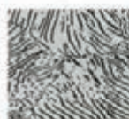
0.8 % C پراولیت
