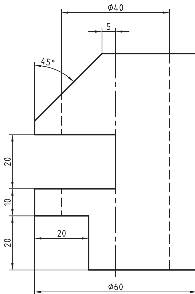
شکل ۳۲-۲ نام: بدنه، جنس: چوب
