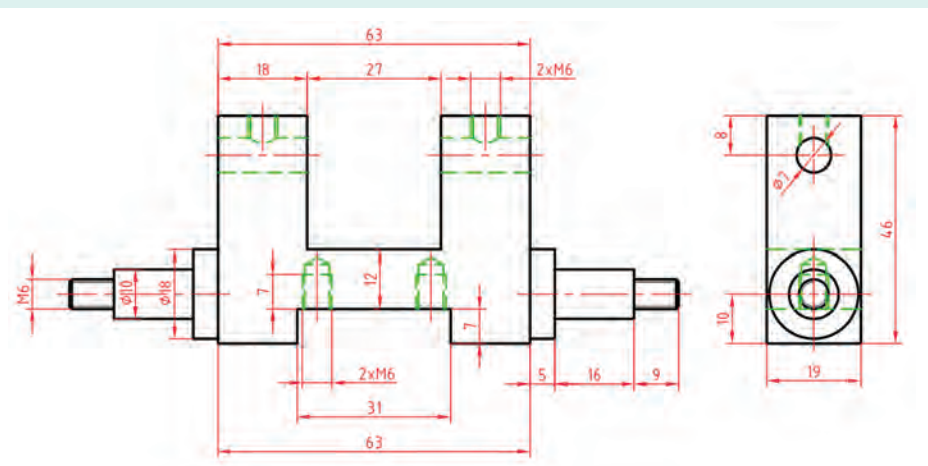
شکل ۲-۲۸- نام: بدنه توپ تزئینی، جنس: آلومینیم
