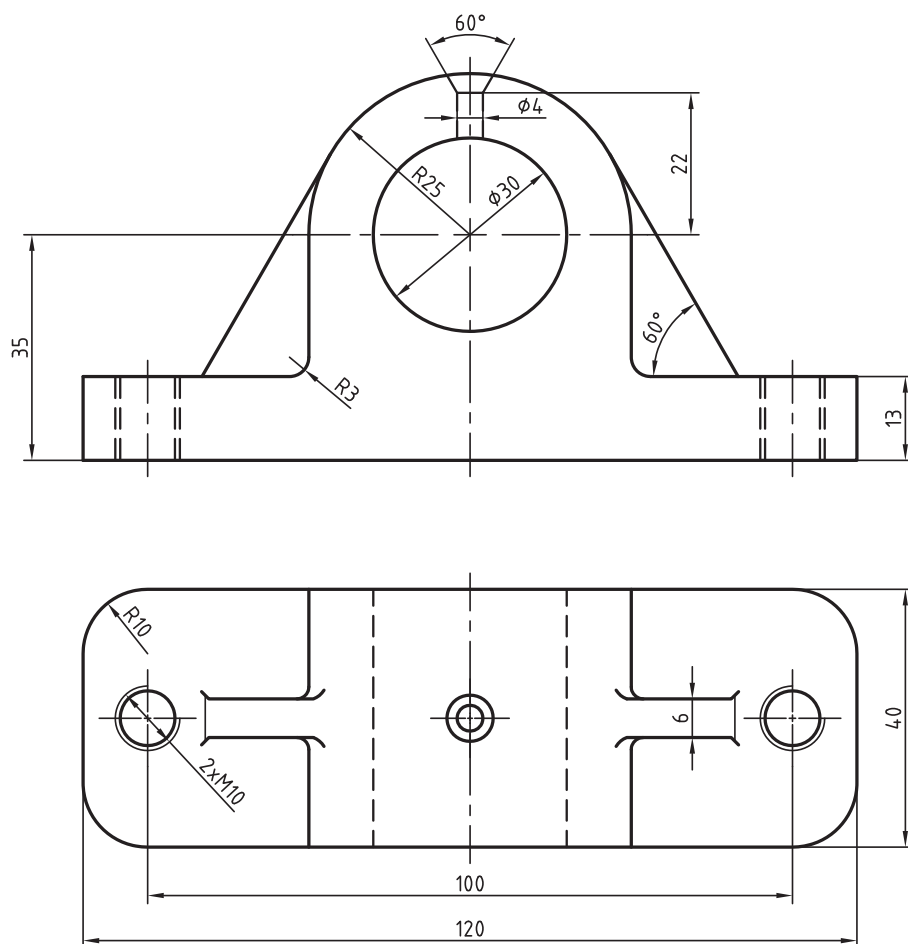
شکل ۲-۲۷- نام: یاتاقان، جنس: چدن
