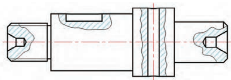
شکل ۳-۶۶- محور فولادی
