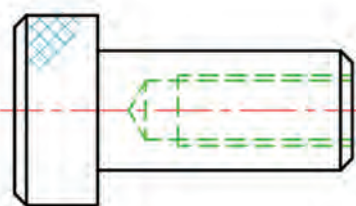
درپوش مخصوص - برنز
