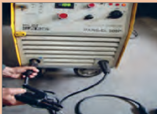
شکل ۴۰- اتصال انبرها
