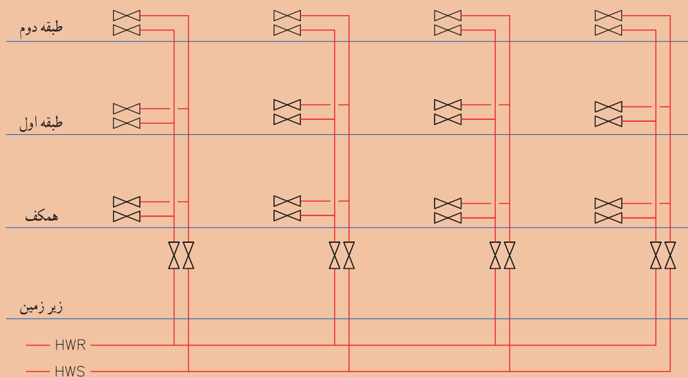
شکل ۱۷- نشت یابی رایزرها رفت و برگشت به تفکیک
