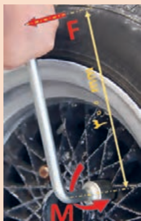
شکل ۵-۱۸- باز کردن پیچ چرخ خودرو توسط آچار چرخ
