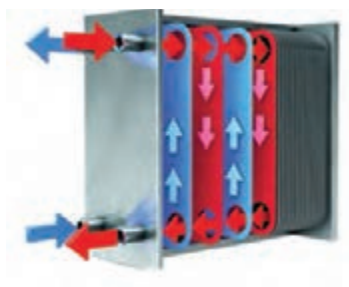
مبدل صفحه‌ای
