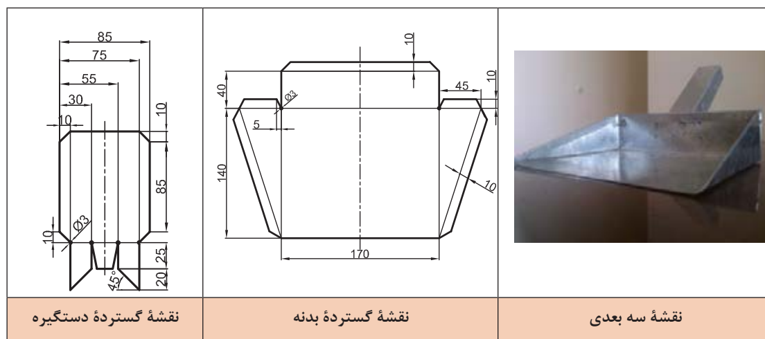
شکل ۱-۵- نقشه خاک‌انداز
