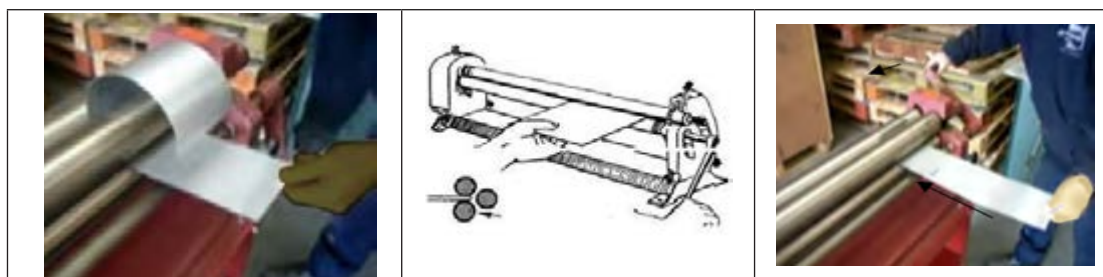
شکل ۳۱-۱- عملکرد دستگاه های خم کن
